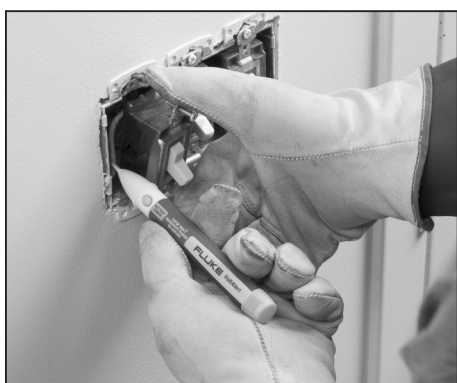
Fluke 2 AC VoltAlert
